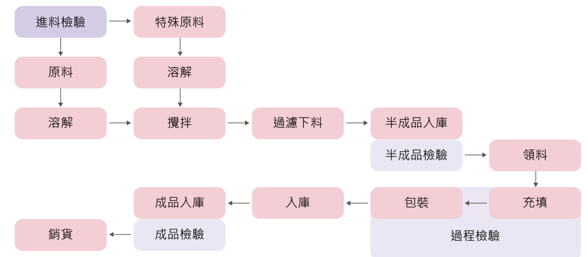
一般液態單元生產工序流程
